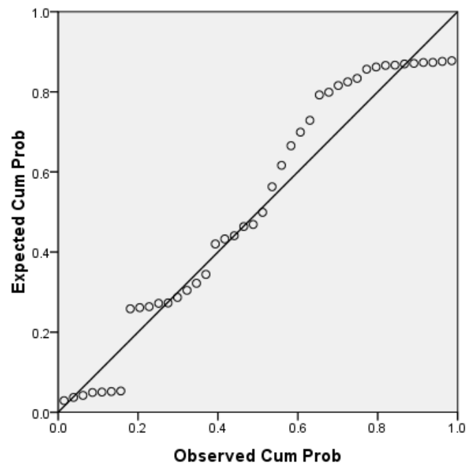
Normal P-P Plot of PEMBIAYAAN YANG DIBERIKAN
